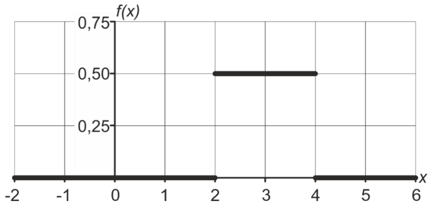
Рис. 2.6. Графік диференціальної функції (закон рівномірної щільності)
