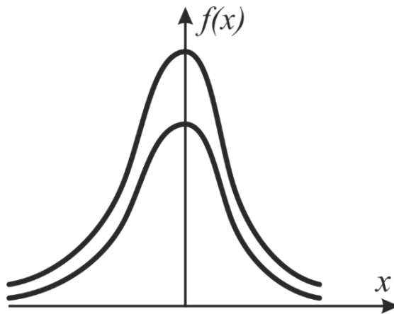
Рис. 5.9. Щільність розподілу закону Стюдента
