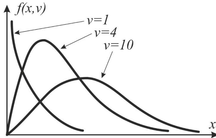
Рис. 5.8. Щільність розподілу закону \chi^2 при різних значеннях параметру v Можна показати, що
