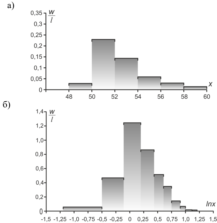
Рис. 5.4. Гістограма відносних частот:
